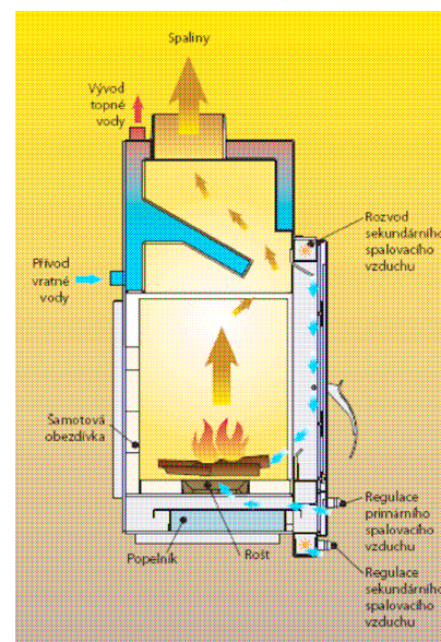
Princíp fungovania teplovodného výmenníka
